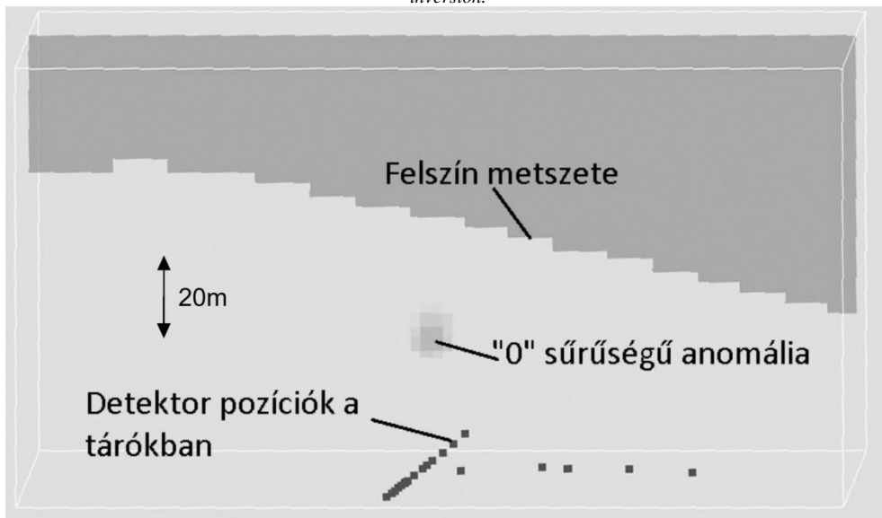
10. ábra: Az anomália képe egy a fő táróra merőleges metszeten.
