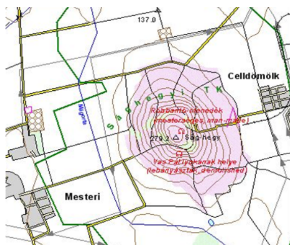
3. ábra A Vas Pál lyukának feltételezett helye (forrás: http://geogr.elte.hu/nonkarstic ) Fig.3. The hypothetical location of the Vas Pál Hole (source: http://geogr.elte.hu/nonkarstic )
