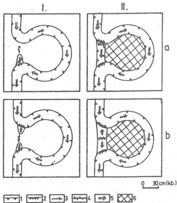
8. ábra: Karros tanuhegyek kialakulása kanyarulat állefejeződésével egy (a), két (b) mellékvályú regressziója esetén Jelmagyarázat: 1. I. típusú vályú, 2. lépcső, 3. vályúvég hátrálásának iránya, 4. vályútalp vízváltzó, 5. I. típusú vályú talpának dőlésiránya, 6. tanuhegy, I. kezdeti állapot, II. kifejezett állapot Figure 8: Developing of karren mesas with pseudocapturing of bends in the case of regression of 1 (a) or 2 (b) ancillary rinnen Legends: 1. I. type karren rinnen, 2. escarpment, 3. direction of withdrawal of rinnen end, 4. rinnen bottom drainage, 5. direction of grade of I. type karren rinnen bottom, 6. mesa I. starting condition, II. full developed condition
