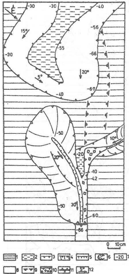
18. ábra: Az "E" jelű karros térszínrészlet morfológiai térképe Jelmagyarázai: 1. a térképezeti térszínrészlet határoló nem, vagy kismértékben karrosodott térszín, 2. felszigethegy, 3. I. típusú vályú (függőleges oldalú) 4. I. típusú vályú (lankás oldalú), 5. III. típusú vályú, 6. függőleges és lankás oldalú madáritató maradvány, 7. vályú és madáritató mélységadattal cm-ben (mélységadat ott került feltüntetésre, ahol az aljzat mélységének mérése történt a peremhez képest), 8. jedőüledék nélküli vályútalp, 9. karbarlang, 10. felnyílásos karrvályú, 11. karrvályú sziklahíd, 12. vályútalp dőlésének iránya és dőlésszö- ge
