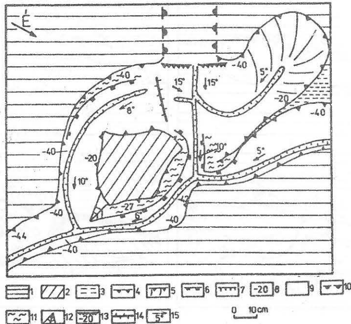
14. ábra: A "C" jelű karros térszínrészlet morfológiai térképe Jelmagyarázat: 1. a térképezett térszínrészlet határoló nem, vagy kisméretűben karrosodott térszínrészlet, 2. szigethegy, 3. felszigethegy, 4. I. típusú vályú (függőleges oldalú), 5. I. típusú vályú (lankás oldalú), 6. II. típusú vályú (függőleges oldalú), 7. III. típusú vályú, 8. vályú mélységadata cm-ben (mélységadat helye ott került feltüntetésre, ahol az aljzat mélységének mérése történt a peremhez képest), 9. fedőüledék mentes vályútalp, 10. karrbarlang, 11. terasz, teraszmaradvány, 12. szoknya, 13. lépcső mélységadattal, cm-ben, 14. vályútalp vízvázlat, 15. vályútalp dőlésének iránya és lejtésszöge
