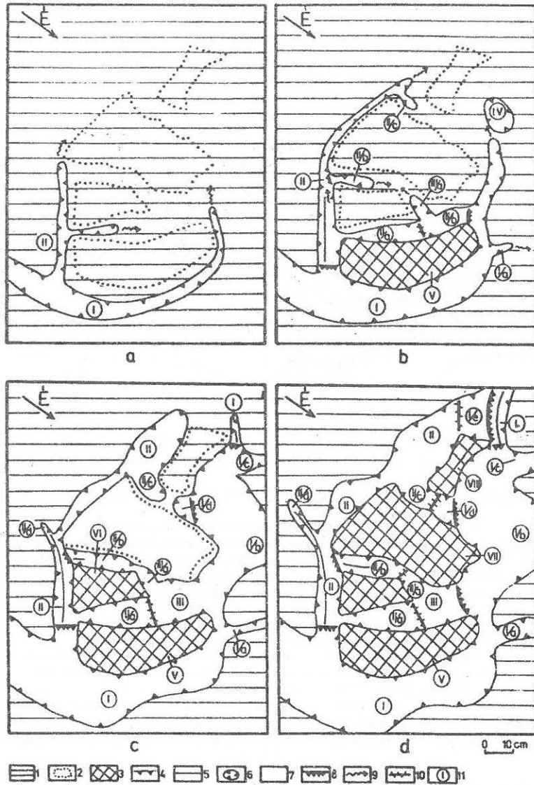
11. ábra: Az "A" jelű karros térszínrészlet kioldódástörténete
