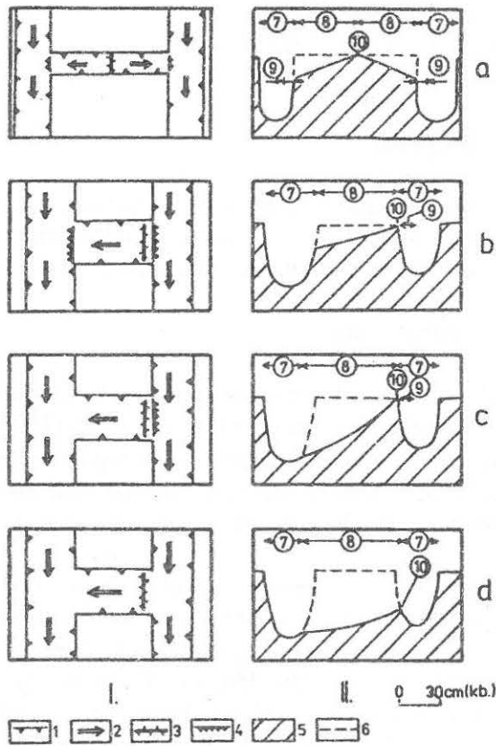
2. ábra: Vályóvég találkozás (a) és állefejeződés (b, c, d) Jelmagyarázat: 1. I. típusú vályú, 2. I. típusú vályú talpának dőlésiránya, 3. vályútalp vízváltzó, 4. lépcső, 5. karrosodó kőzet, 6. vályúbemélyülés előtti térszín, 7. fővályú, 8. regresszáló mellékvályú, 9. lépcső, 10. vályútalp vízváltzó I. felülnézet II. oldalnézet (metszetek az összekapcsolódó illetve a lefejezést végző vályúk mentén), a hátráló vályúvégek összekapcsolódnak (a), a lefejező vályú egyenletesen mélyül (b) a lefejező vályú hátrál (c) a lefejező vályú a fővályú talpáig mélyül (d) Figure 2: Meeting of rinnen (a) ends and pseudocapturing (b, c, d) Legends: 1. I. type karren rinnen, 2. direction of dip of I. type karren rinnen bottom, 3. rinnen bottom drainage, 4. escarpment, 5. rock developing karren, 6. ground surface before rinnen depression, 7. main rinnen, 8. regressive ancillary rinnen, 9. escarpment, 10. rinnen bottom drainage I. view from above II. side view (segments by the side of rinnen doing capturing), the retrogressive rinnen ends join together (a), the capturing rinnen deepens consistently (b), the capturing rinnen withdraws (c), the capturing rinnen deepens to the bottom of main rinnen (d)
