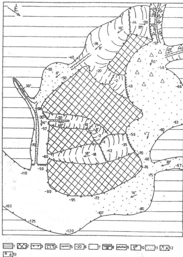
10. ábra: A: "A" jelű térszínrészlet morfológiai térképe
