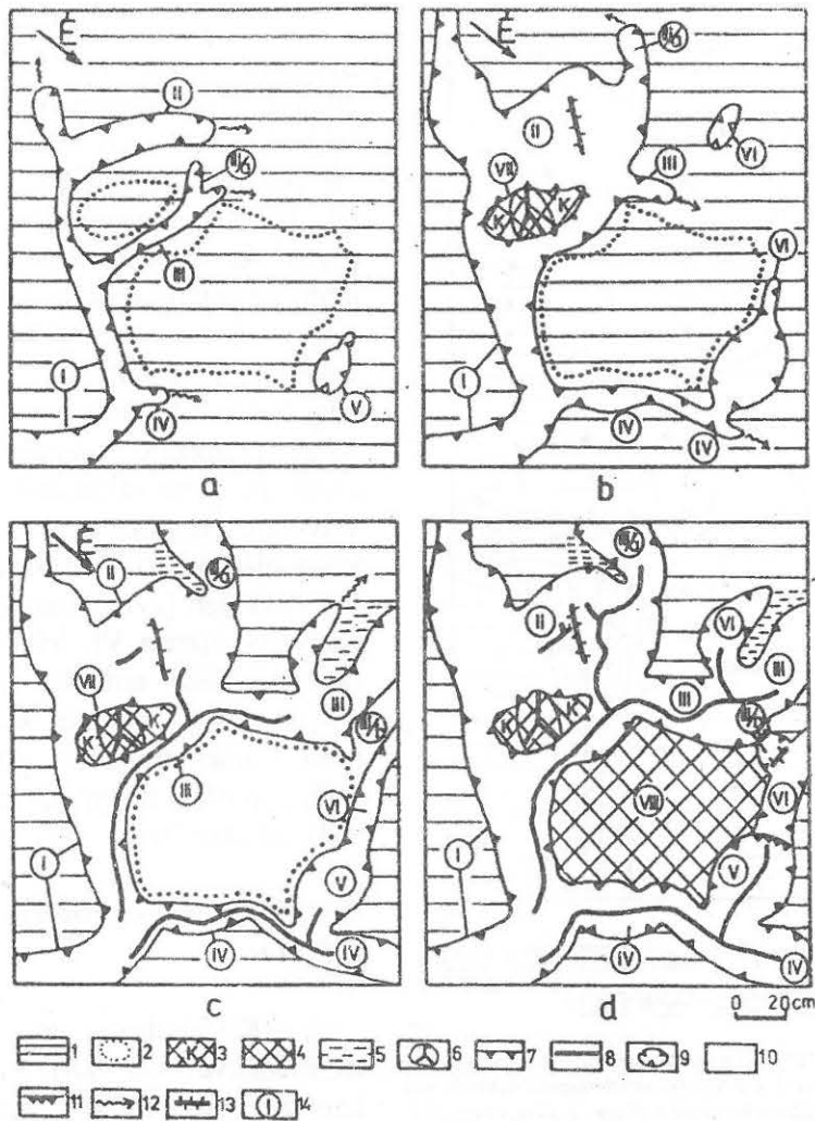
17. ábra: A "D" jelű karros térszínészlet kioldódástörténete
