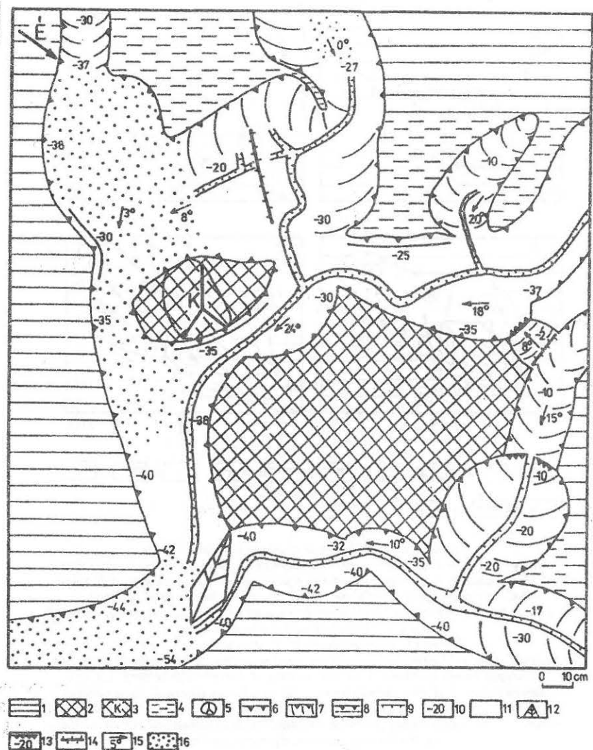
16. ábra: A "D" jelű karros térszínrészlet morfológiai térképe
