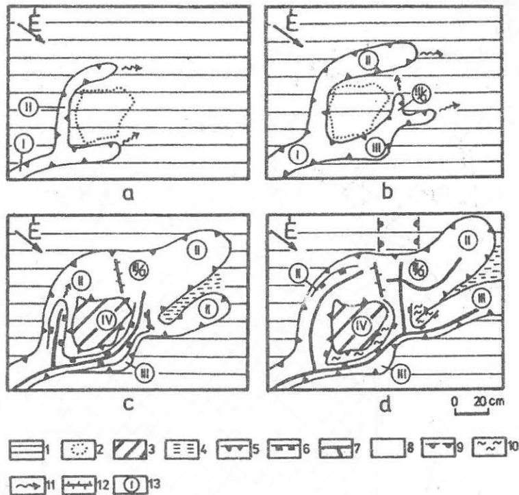
15. ábra: A "C" jelű karros térszínrészlet kioldódástörténete Jelmagyarázat: 1. nem karrosodó, vagy rekonstruálható kariformát még nem hordozó térszín, 2. később kialakuló szigethegy, 3. szigethegy, 4. félszigethegy, 5. I. típusú vályú, 6. II. típusú vályú, 7. III. típusú vályú, 8. fedőüledék nélküli vályútalp, 9. karrbarlang, 10. terasz, 11. vályúvég hátrálásának iránya, 12. vályútalp vízválasztó, 13. karrvályú és szigethegy azonosító jele a. b. c. korábbi állapot, d. jelenlegi állapot
