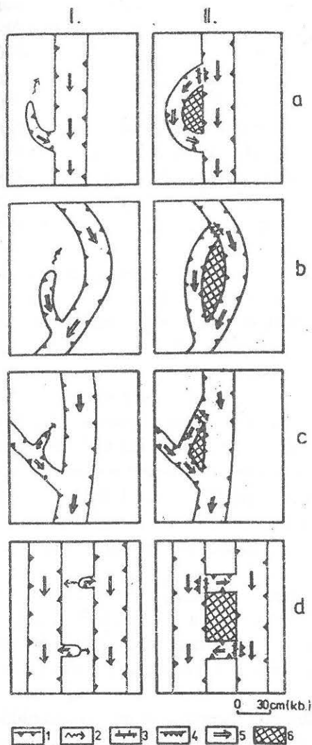
5. ábra: Karros tanuhegyek kialakulása állefejeződésekkel Jelmagyarázat: 1. I. típusú vályú, 2. vályúvég hátrálásának iránya, 3. vályútalp vízváltató, 4. lépcső, 5. I. típusú vályú talpának lejtésiránya, 6. tanuhegy, I. kezdeti állapot, II. kifejlett állapot
