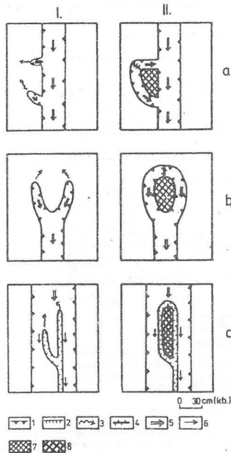
4. ábra: Karros sziget- és tanuhegyek kialakulása vályúvég találkozásokkal
