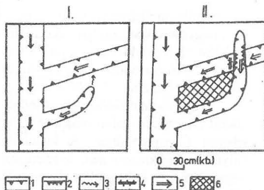
6. ábra: Karros tanuhegy kialakulása igazi lefejeződéssel Jelmagyarázat: 1. I. típusú vályú, 2. lépcső, 3. vályúvég hátrálásának iránya, 4. vályútalpi vízvásztó, 5. I. típusú vályútalpi lejtésének iránya, 6. tanuhegy, I. kezdeti állapot, II. kifejlett állapot.
