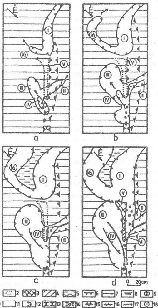
19. ábra: Az "E" jelű karros térszínrészlet kioldódástörténete Jelmagyarázat: 1. nem karrosodó, vagy rekonstruálható karrformát még nem hordozó térszín, 2. később kialakuló sziget- és tamuhegy, 3. tamuhegy, 4. szigethegy, 5. felszigethegy, 6. I. típusú vályú, 7. III. típusú vályú, 8. lépcső, 9. madáritató, 10. roncsolódott madáritató, 11. vályú- és madáritató talp, 12. karrvályú víznyelő, 13. karrbarlang, 14. felnyílásos karrvályú, 15. karrvályú szaklahíd, 16. vályútalp vízválasztó, 17. vályúvég hátrálásának iránya, 18. karrvályú, madáritató és tamuhegy azonosító jele, a, b, korábbi c, jelenlegi, d jövőbeni állapot Figure 19: Solution history of "E" ground surface part Legends: 1. do not karren surface, or there is not reconstructable karren forms, 2. later developed karren inselberg and mesa, 3. mesa, 4. karren inselberg, 5. karren haifinselberg, 6. I. type karren rinnen, 7. III. type karren rinnen, 8. escarpment, 9. kamenitza, 10. destructive kamenitza, 11. rinnen and kamenitza bottom, 12. rinnen sink, 13. karren cave, 14. opening rinnen, 15. rinnen arch, 16. rinnen bottom drainage, 17. direction of withdrawal of rinnen end, 18. identity sign of rinnen, kamenitza and mesa (a, b, former condition, c present condition, d condition in the future)
