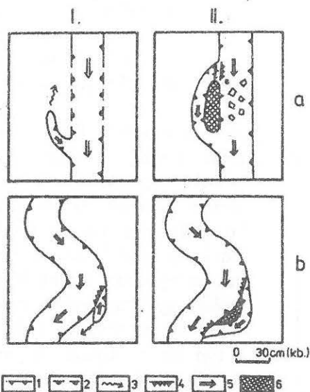
7. ábra: Karros tanuhegy kialakulása karrbarlang felnyílása (a) és antiregressziós vályú (b) képződése esetén Jelmagyarázat: 1. I. típusú vályú, 2. karrbarlang, 3. vályúvég hátrálásának iránya, 4. lépcső, 5. I. típusú vályú talpának lejtés iránya, 6. tanuhegy I. kezdeti állapot, II. kifejeleti állapot Figure 7: Developing of karren mesas after opening up the karren cave (a) and developing of antiregression rinnen (b) Legends: 1. I. type karren rinnen, 2. karren cave, 3. direction of withdrawal of rinnen end, 4. escarpment, 5. direction of grade of I. type karren rinnen bottom, 6. mesa I. starting condition, II. full developed condition
